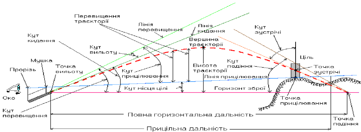
Мал. 3. Елементи траєкторії.
