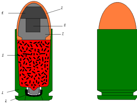
Мал. 3. Розріз 9 мм пістолетного патрона та його загальний вигляд:
