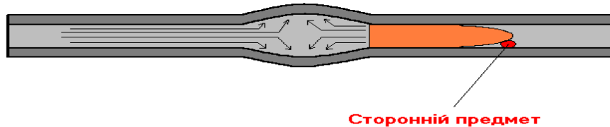
Мал. 2 Роздуття каналу ствола.
