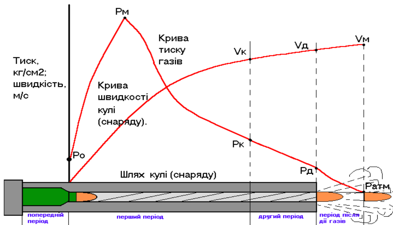
Мал. 1. Періоди пострілу.
